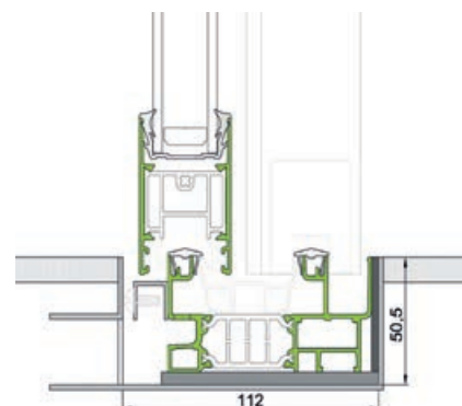
Raíl adaptado a PMR. Corredera 2 railes con marco inferior empotrado con bandeja inox.
